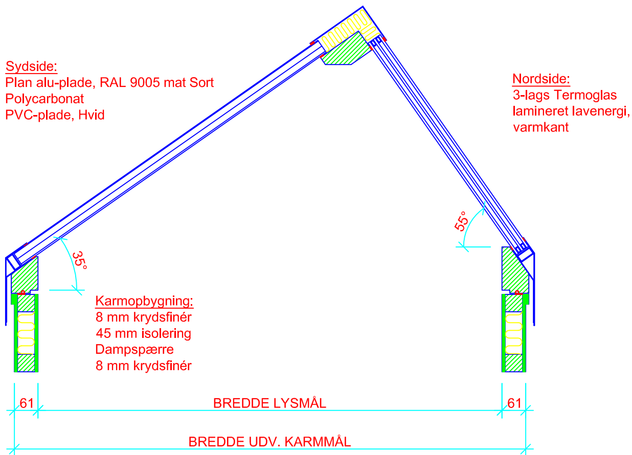
TVÆRSNIT
